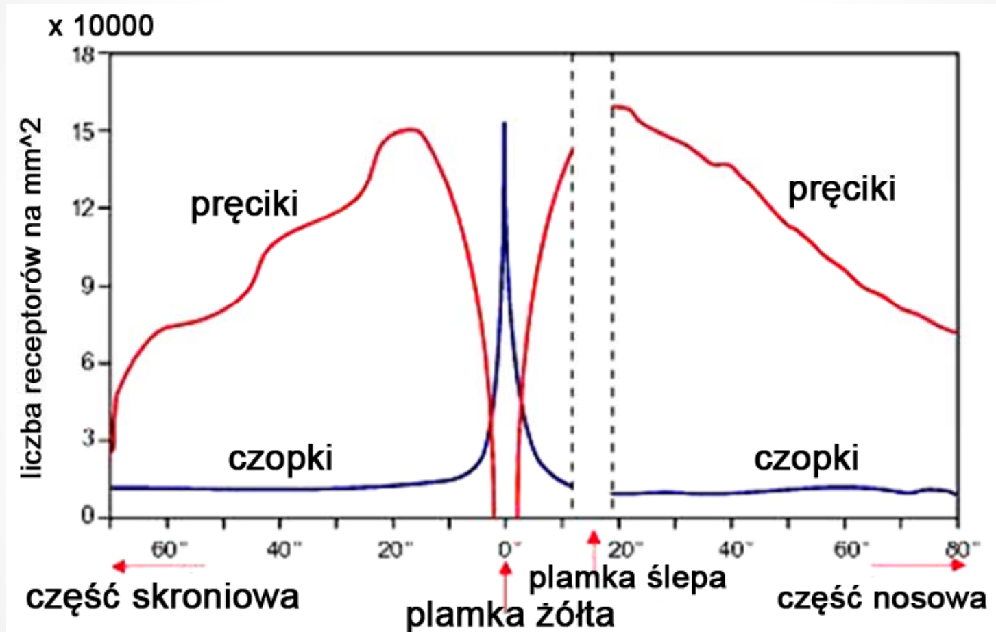
Rys.5 Rozkład pręcików i czopków na siatkówce oka
