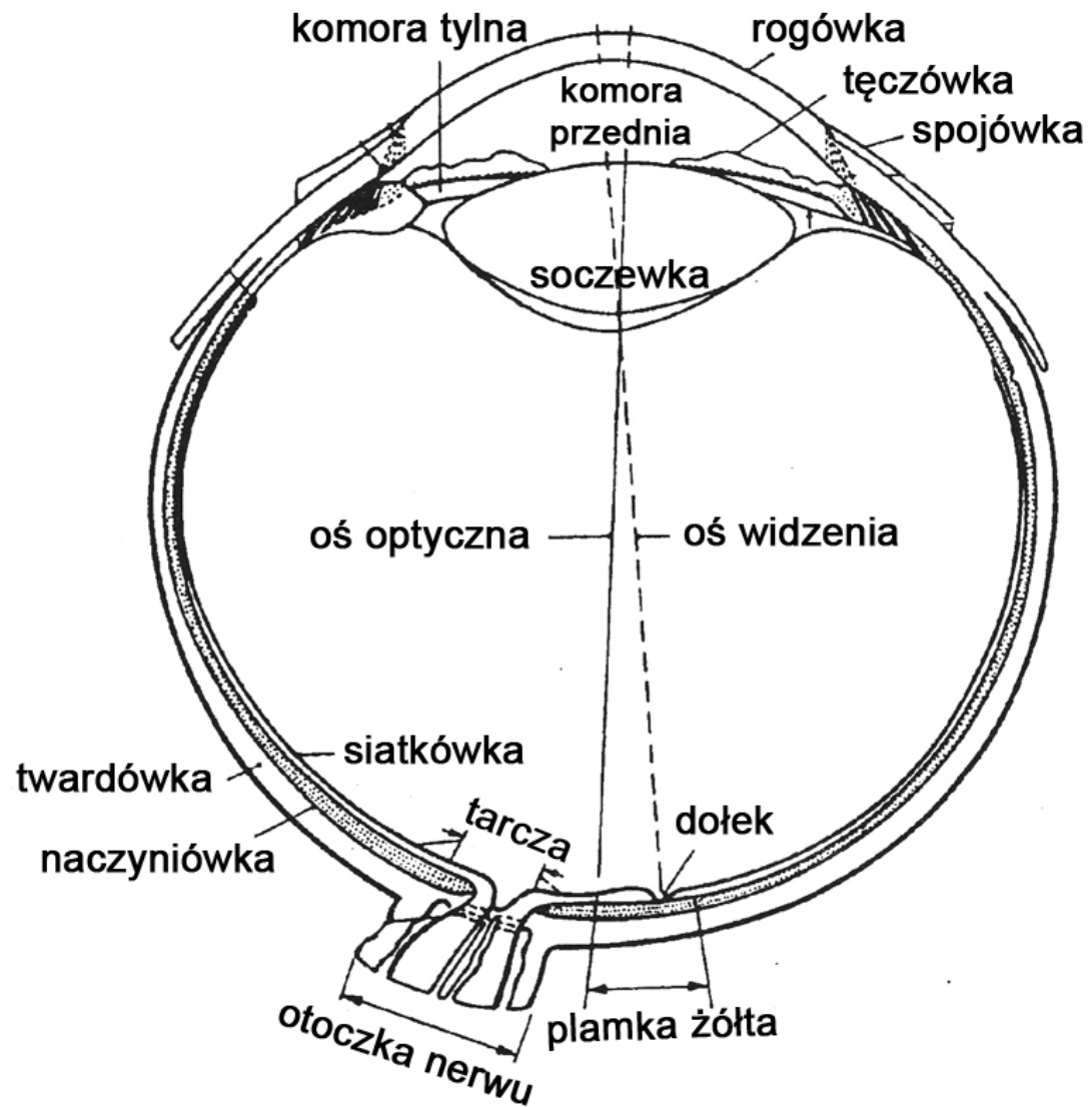
rys. schemat poprzeczny gałki ocznej
