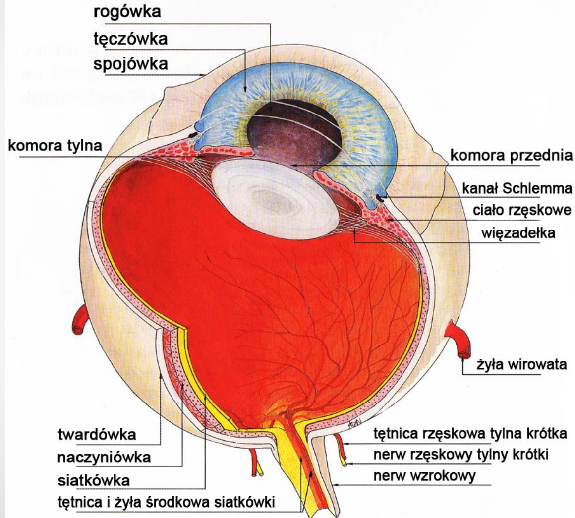
Rys. 4 Schemat budowy oka
