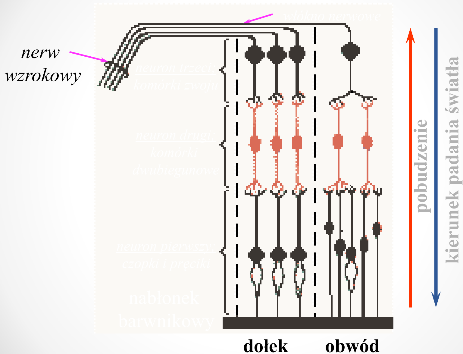
rys. 1. elementy nerwowe siatkówki
