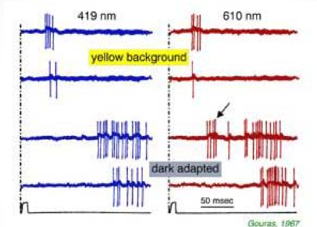
Rys. A. 29 . Porównanie czasu reakcji komórki zwojowej w przypadku stymulacji „preferowanym” przez pręciki (419nm) i czopki (610nm) światłem, przy żółtym tle oraz po adaptacji do ciemności. (źródło: http://195.117.188.199/a4.htm )
